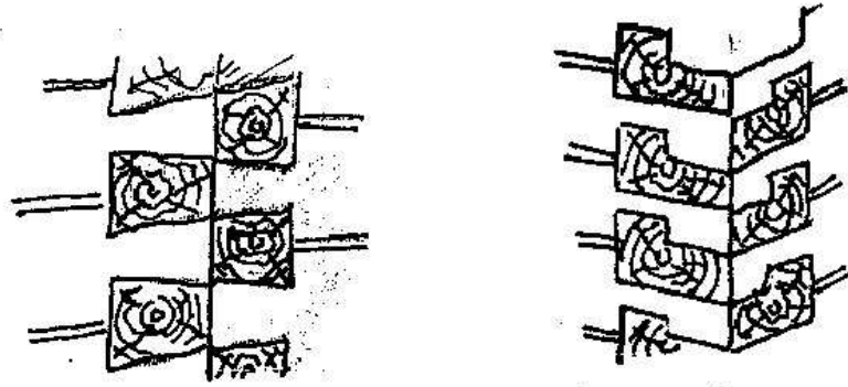
Druhy spojování trámů u roubenek: „na rybinu“ a „na zámek“
